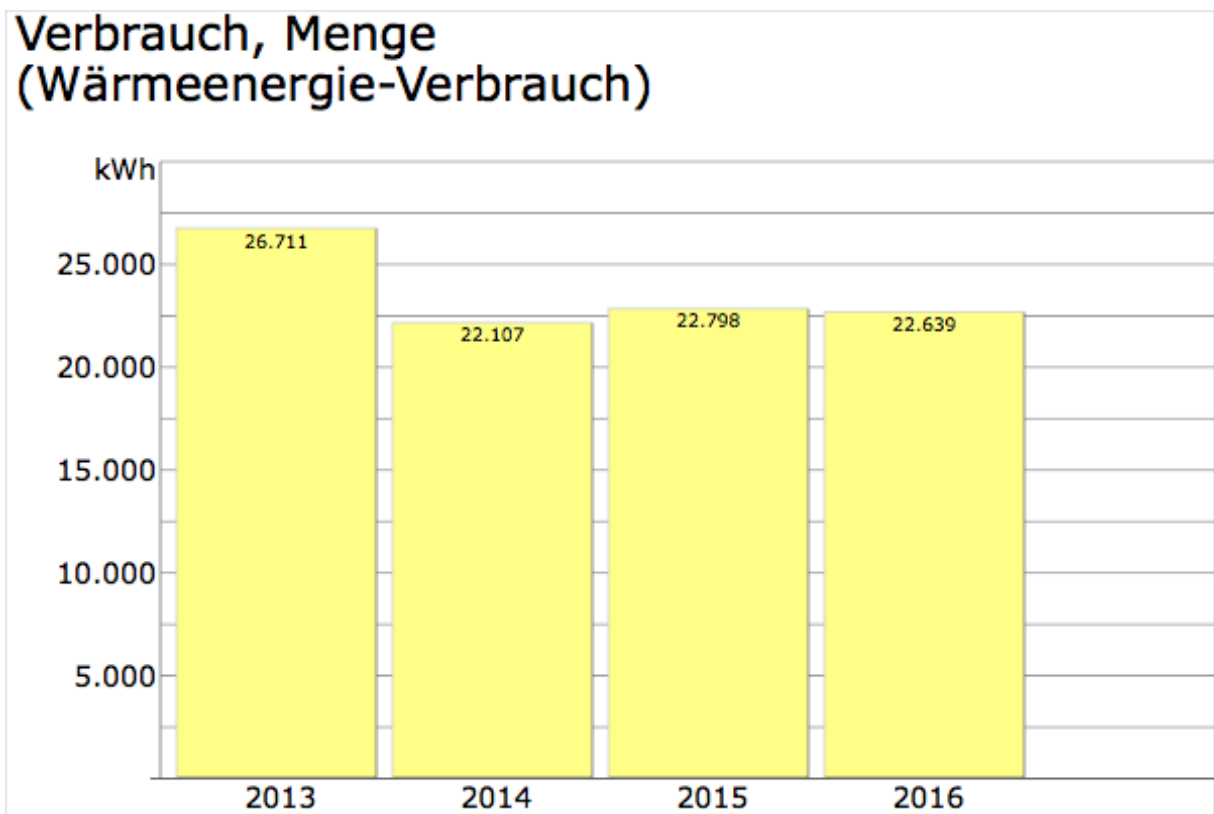
Diagramm Wärmeenergie Paul-Gerhardt-Haus Walstedde (tatsächliche Verbrauchswerte)
