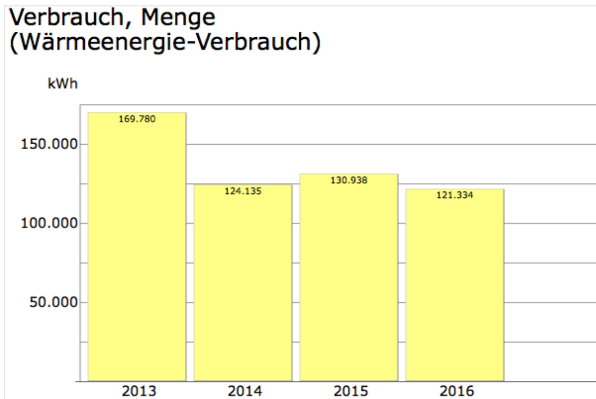
Diagramm Wärmeenergie Pauluskirche (tatsächliche Verbrauchswerte)
